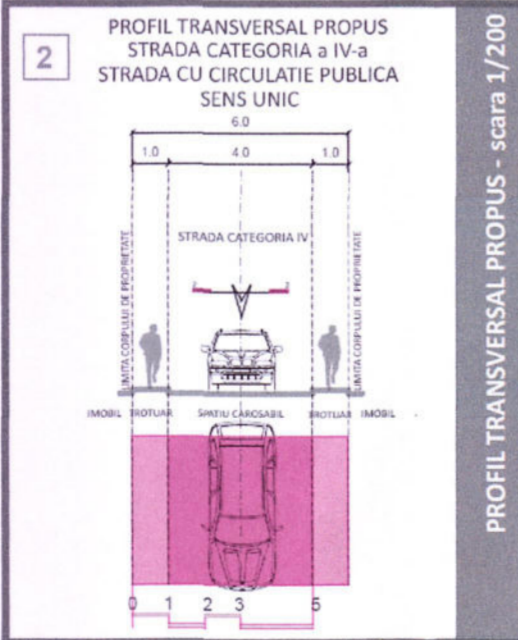
PROFIL STRADAL PROPUȘ ÎN PUZ VIABILIZARE ZONA COLINARĂ BAI A MARE
