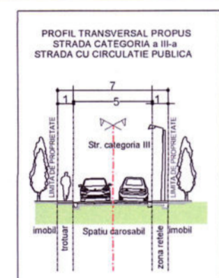
PROFIL STRADAL PROPUȘ 4 - 4
