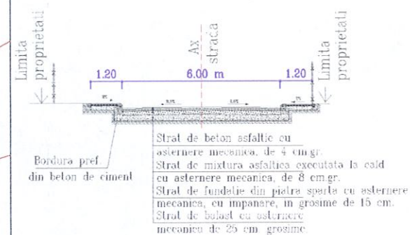
PROFIL TRANSVERSAL A-A str. CHIOARULUI sc 1:200
