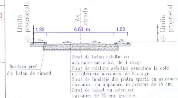
PROFIL TRANSVERSAL B-B str. VRANCEI sc 1:200
