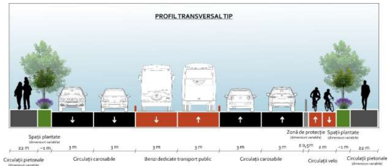
Figură 155 - Profil transversal TIP pentru proiectul Io6
