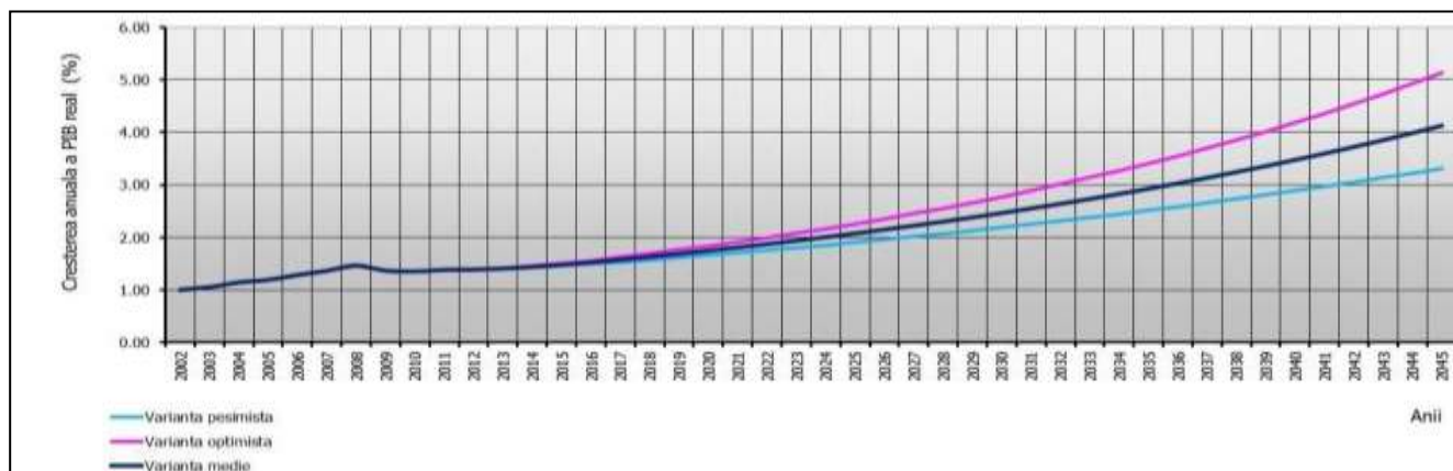
Figură 104 - Prognoza evoluției PIB real până în 2045
