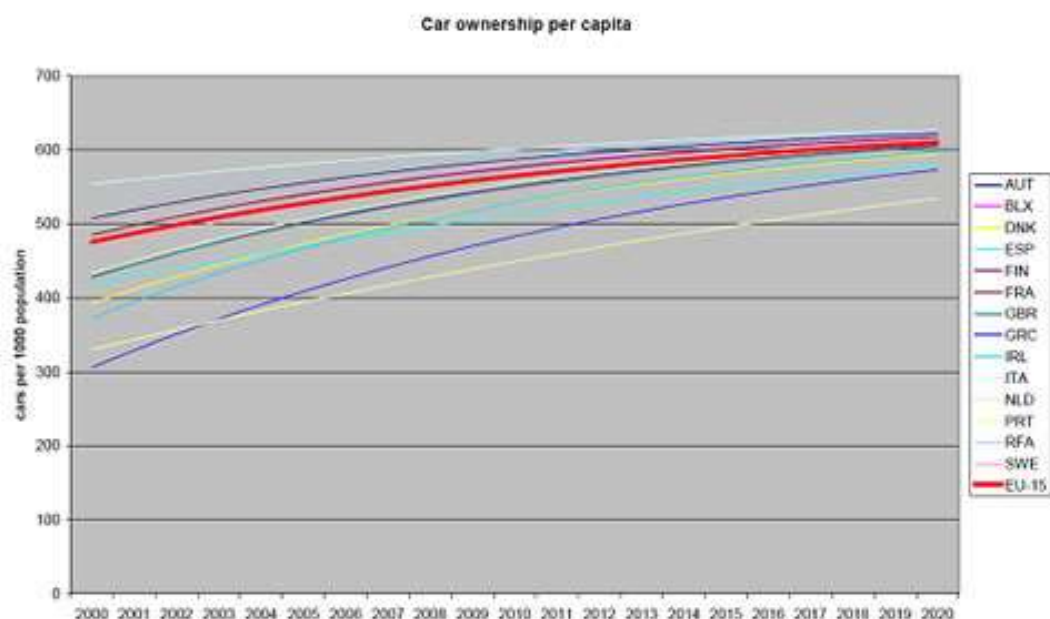
Figură 107 - Prognoza gradului de motorizare pentru țările UE-15; Sursă: Trends in vehicle and fuel technologies - Scenarios for future trends
