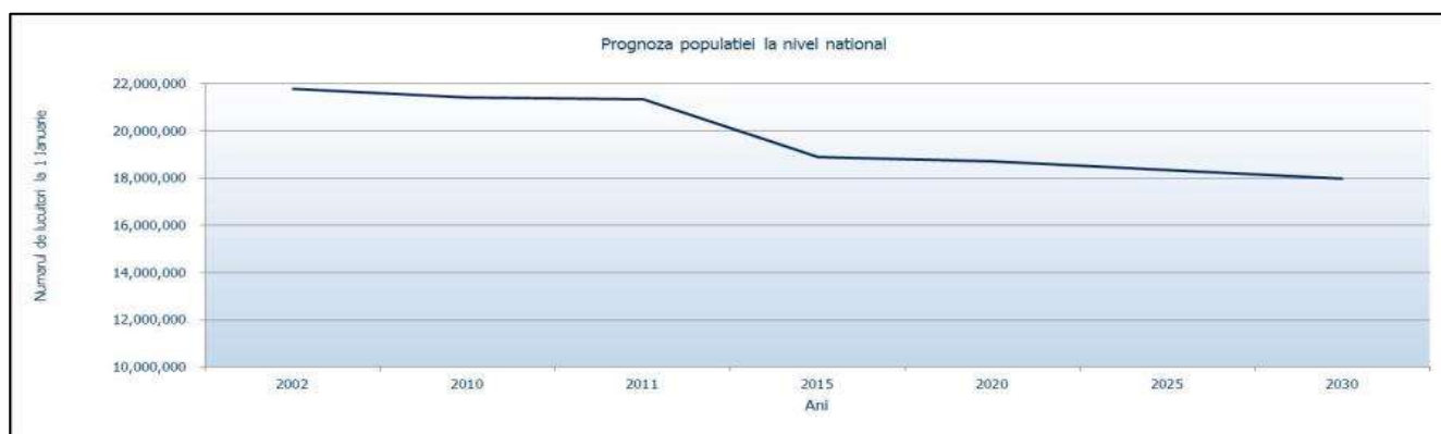
Figură 105 - Prognoza populației până în 2030
