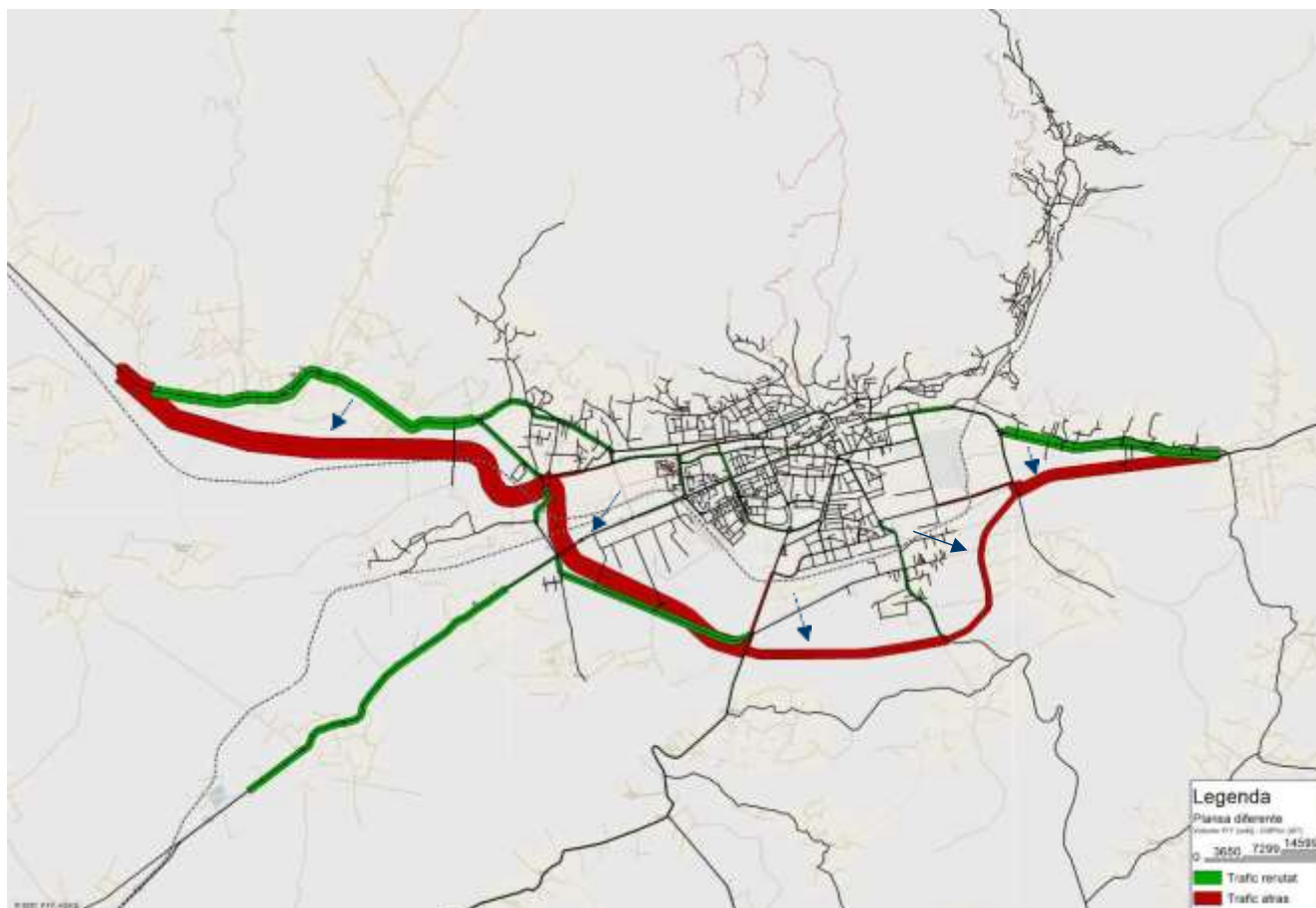
Figură 111 - Planșa diferențe în cazul celor două scenarii testate – „cu proiect” vs „fără proiect”
