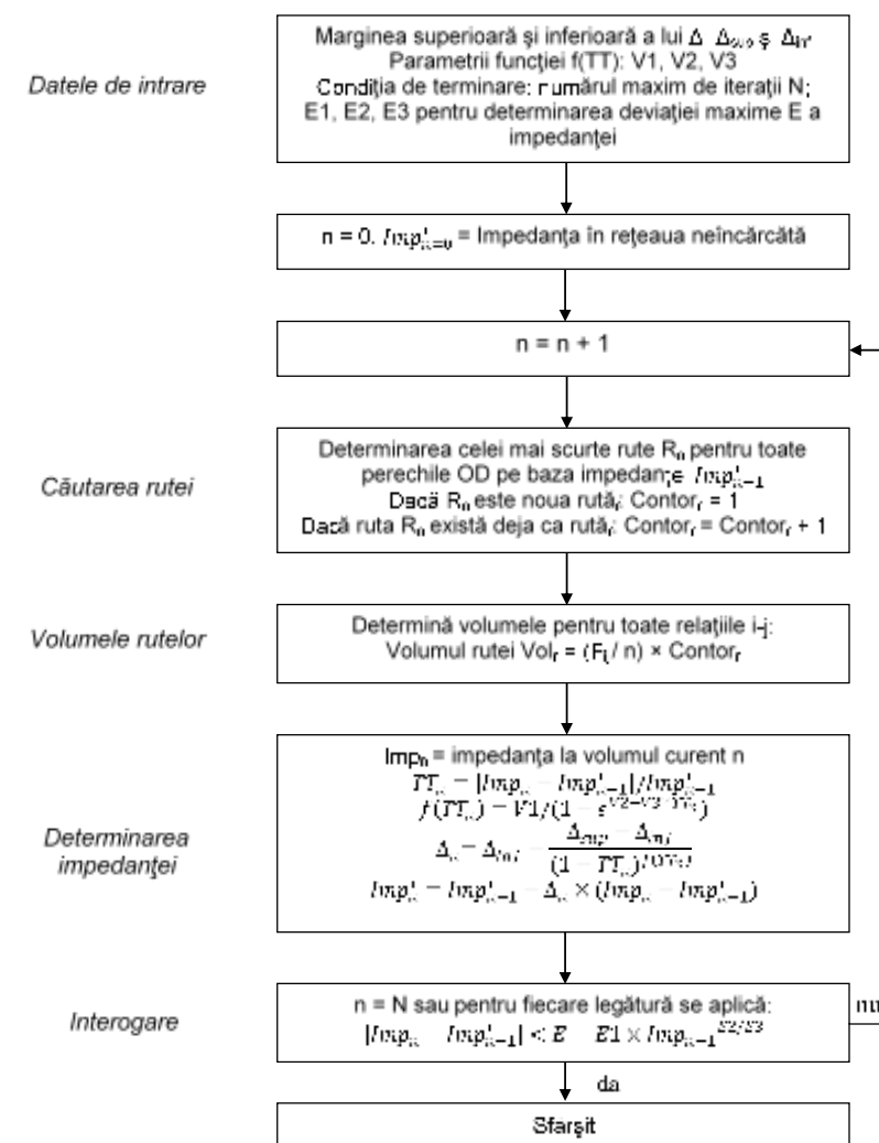
Figură 99 - Schema logică a metodei "Echilibru-Lohse" de afectare pe itinerarii
